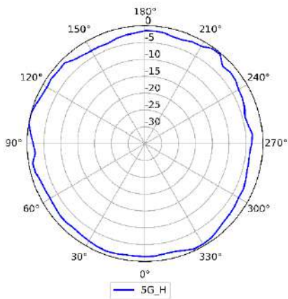
5GHz (Horizontal)
